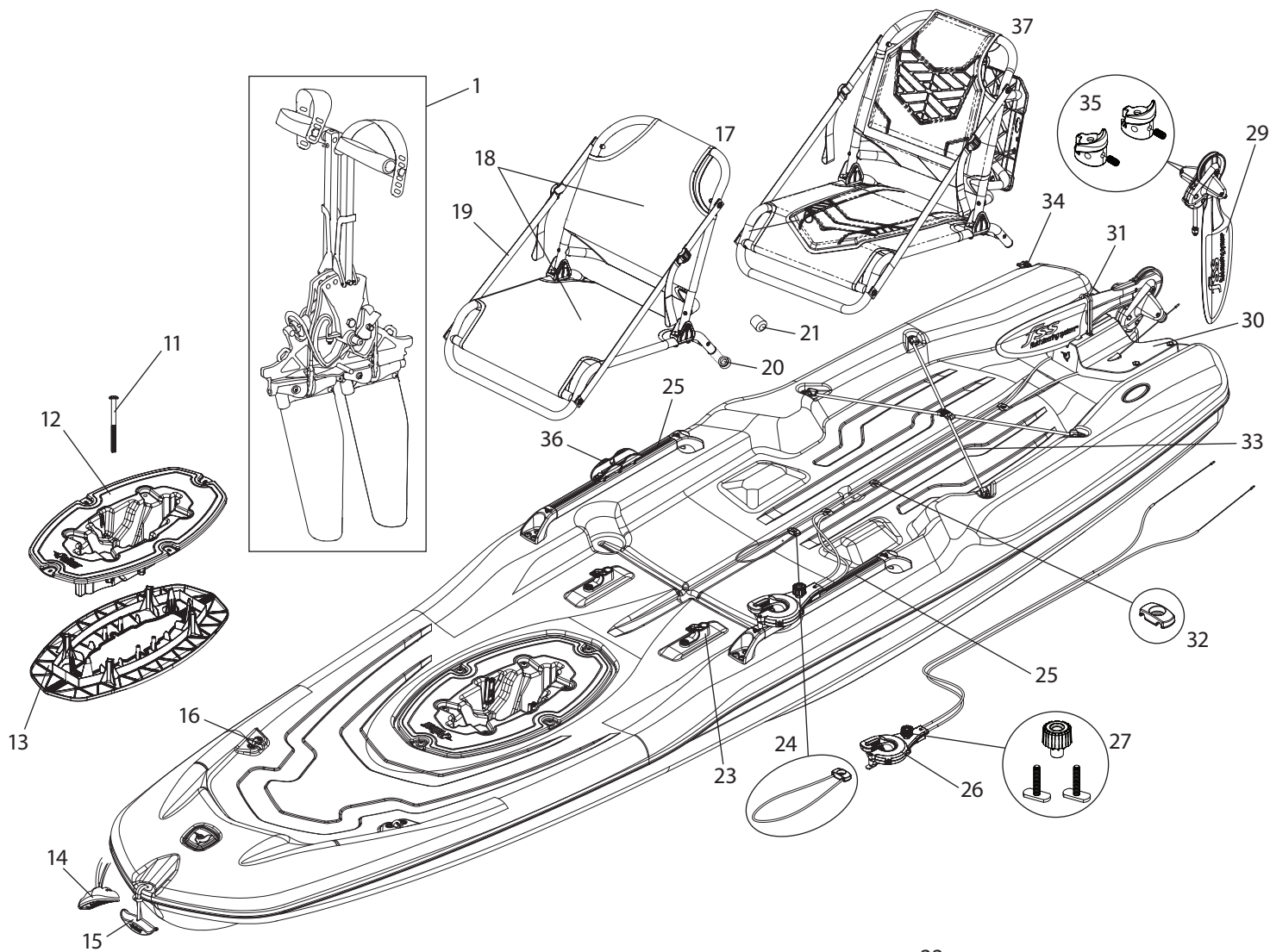
ERGOCAST XP™ & ERGOBOOST GT™ hardware kit - Ensemble de quincaillerie ERGOCAST XP™ et ERGOBOOST GT™
